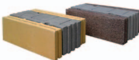
MONOS (facciavista) "U" = 0,33 W/m²K
