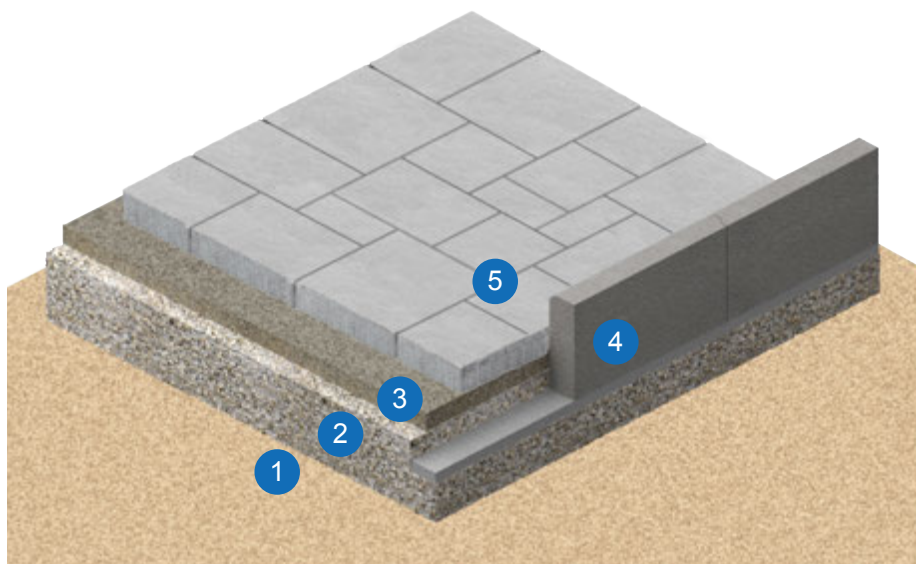
1) Suolo di fondazione; 2) Massicciata; 3) Allettamento di posa; 4) Cordolo di contenimento; 5) Rivestimento (masselli)
